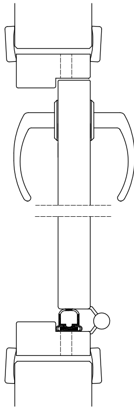
Infällt klämskydd : brandklass upp till E30/EI30 och ljudklass upp till 30dB
