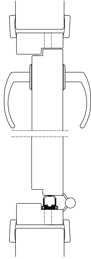
Infällt klämskydd : brandklass upp till EI30 och ljudklass upp till 30 dB
