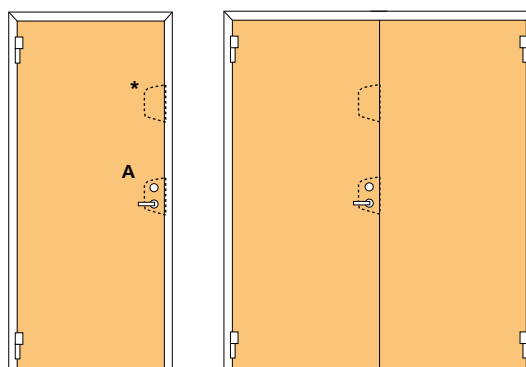
A. Låshus Assa Evolution 310 * Urtag för extra lås
