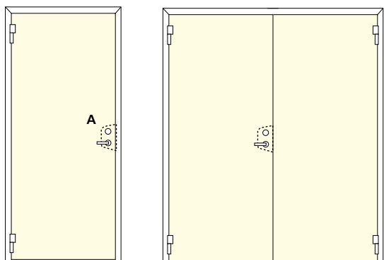
A. Låshus Assa Evolution 310
