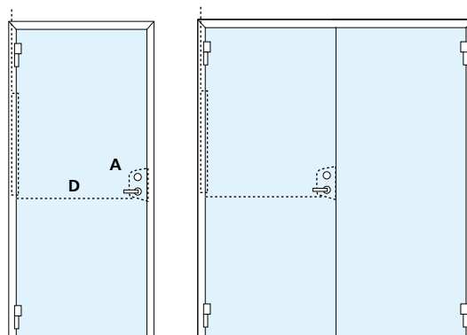
A. Låshus Assa Evolution 410 med microbrytare D. Urtag för karmöverföring, rördragning
