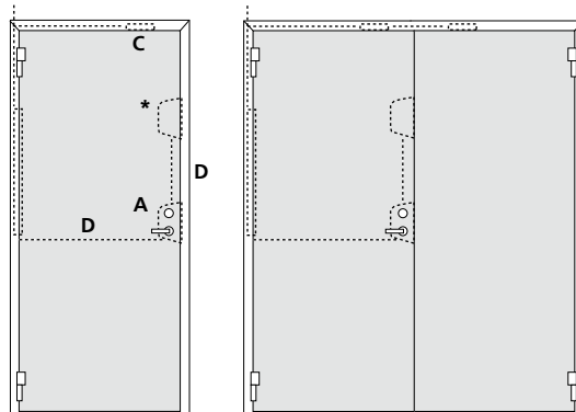
A. Låshus Assa Evolution 310 C. Magnetkontakt D. Urtag för karmöverföring, rördragning * Urtag för extra lås
