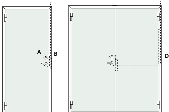
A. Låshus Assa Evolution 222 B. Urtag för el-slutbleck D. Urtag för karmöverföring, rördragning
