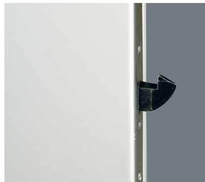
Säkerhetsdörr S23 har ett flerpunktslås där huvudlåset kompletteras med hakreglar upp- och nedtill.
