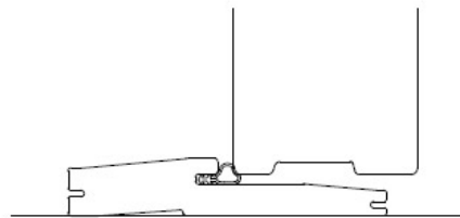
Composieten dorpel
