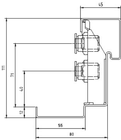
Kozijn 41
