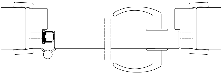
Infällt klämskydd
