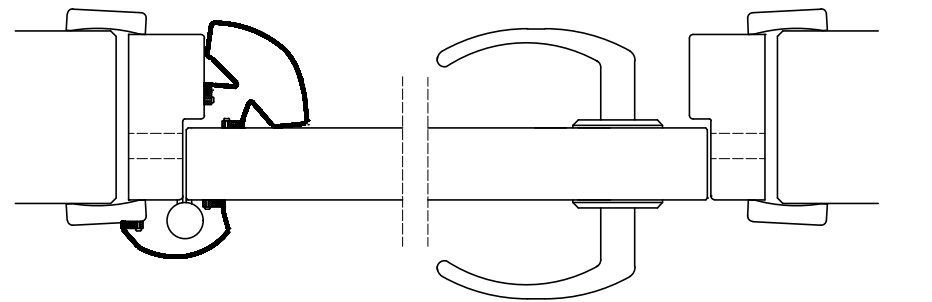
Utanpåliggande klämskydd
