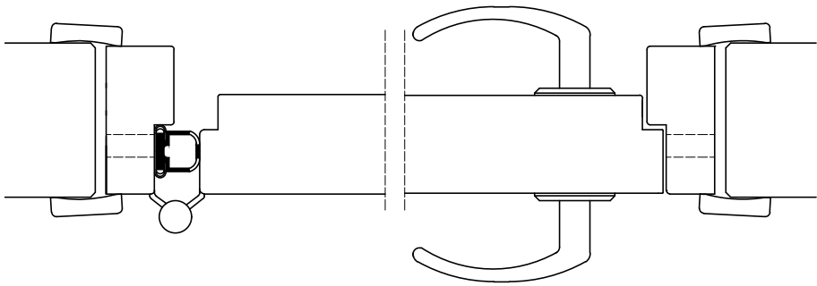
Infällt klämskydd
