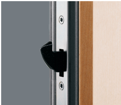
Säkerhetsdörr D43 har ett flerpunktslås där huvudlåset kompletteras med hakreglar upp- och nedtill.
